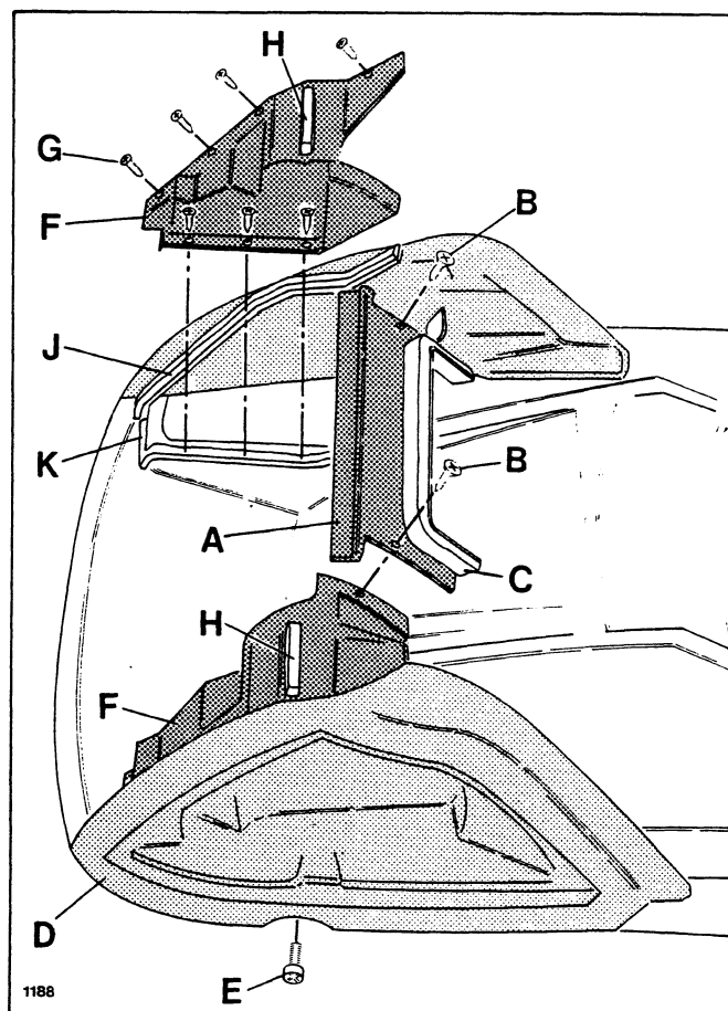
Leuchtengehäuse und Luftkanal
