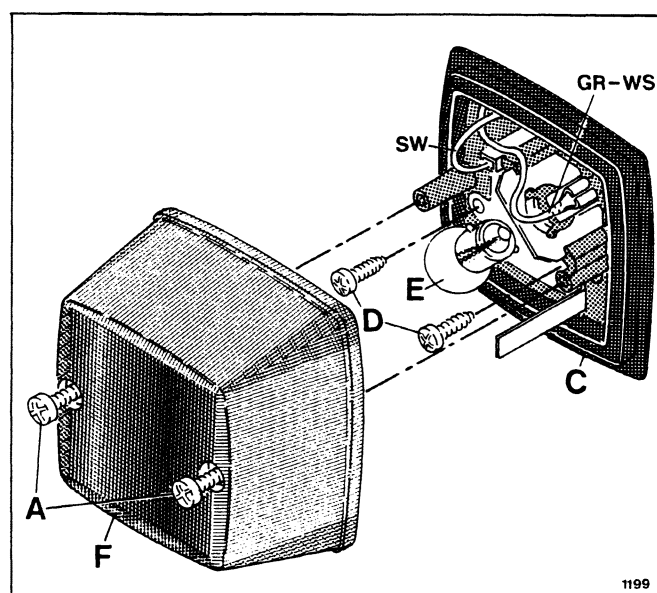
Rückfahrleuchte
